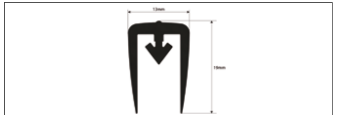
RubberDwarsSysteem2-3-4.png
