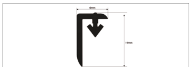
RubberMuurSysteem1-2-3-4.png
